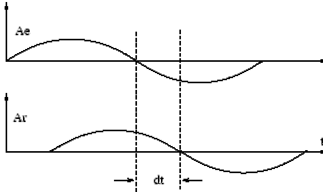
FIGURA 2 - Princípio de medição de tempo no sistema de onda contínua
