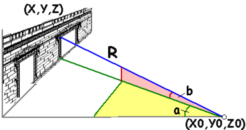
FIGURA 3 - Geometria da varredura laser
