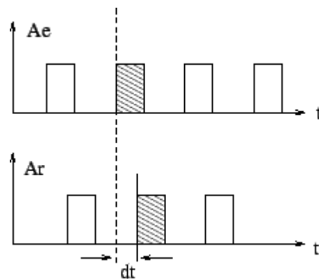
FIGURA 1 - Princípio de medição de tempo no sistema de pulso (Adaptado de Wehr & Lohr [1999])
